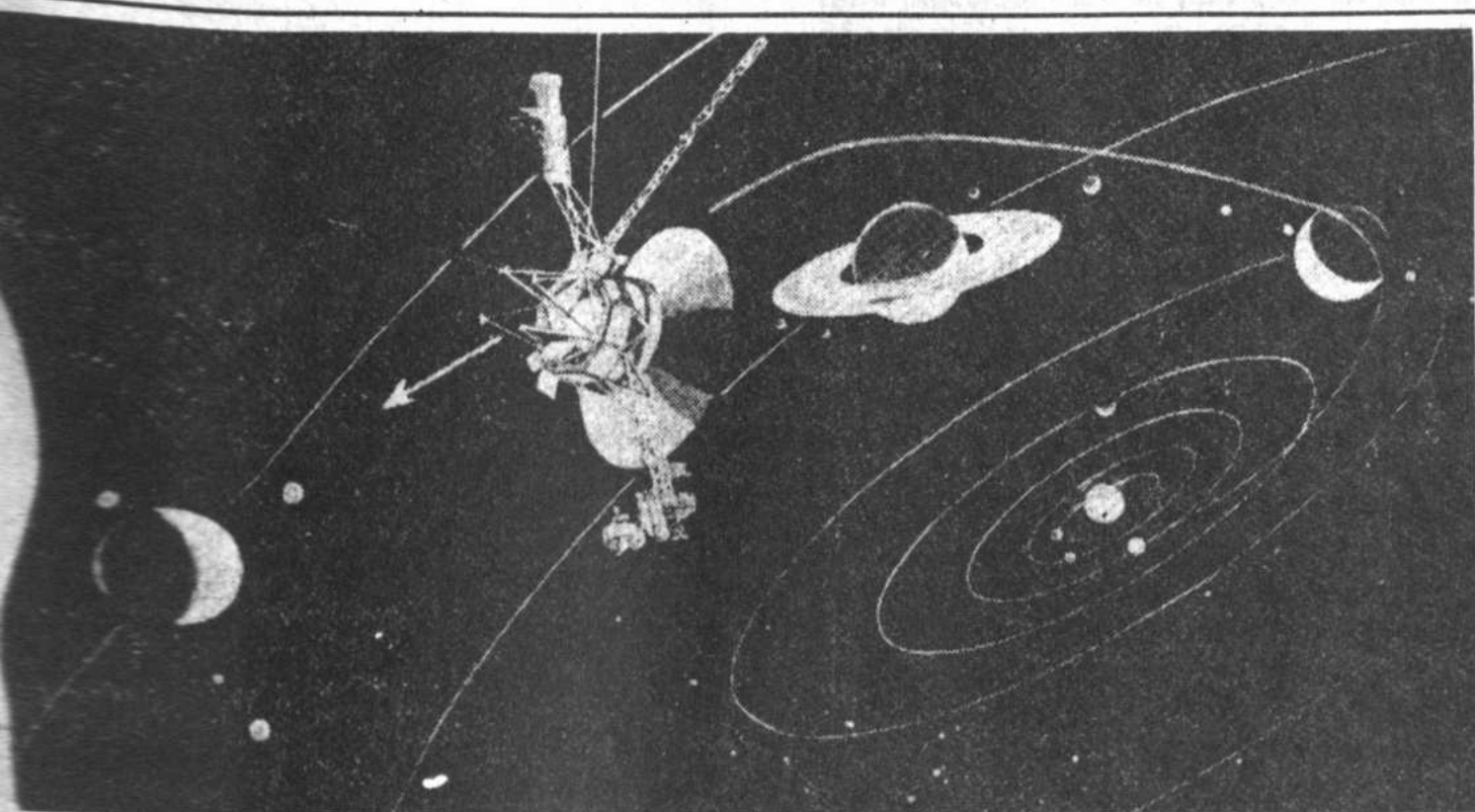
DIBUJO QUE MUESTRA EL ACERCAMIENTO DE LA NAVE VOYAGER 2 A URANO
