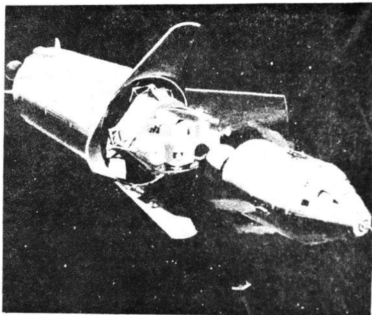
5.— Los astronautas en el Módulo de Mando (al cual está unido el Módulo de Servicio) se separan de la cubierta protectora (de la cual se ve sobresalir el Módulo Lunar). El cohete de la tercera sección, escasamente visible, está conectado detrás de la cubierta del Módulo Lunar.
