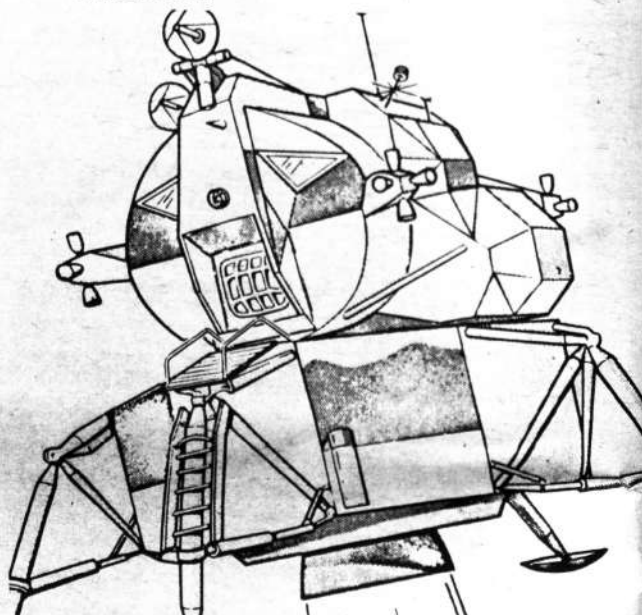
10.— Mientras mantienen al Módulo Lunar en órbita terrestre durante toda la prueba, los astronautas del Apolo-9 simulan un aterrizaje en la Luna. Encienden el motor de descenso que se usará en el aterrizaje en la Luna, y después activan el motor de ascenso que se usará en el lanzamiento desde la Luna.
