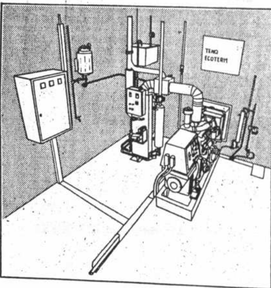
Montaje para producir energía eléctrica y vapor de agua caliente
