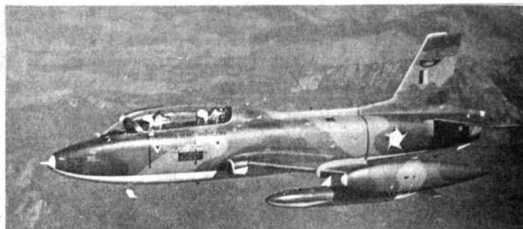
EMB-326 GB XAVANTE Es considerado como la mejor elección en términos de costo/efectividad para efectos de entrenamiento y apoyo aéreo. La velocidad de operación de este avión, llega a Mach 0.82. Puede transportar cargas externas colgadas bajo las alas para vuelos de reconocimiento y ataque.
