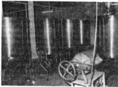
VISTA PARCIAL DE LA SALA DE JARABES. Los recipientes son destinados a recibir los preparados de jarabe para cada uno de los sabores de productos Sucre y Pepsi Cola.
