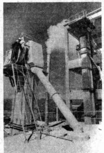
SISTEMA PRECALENTADOR.- La foto muestra el sistema de precalentador "Wedag" de uno de los hornos rotatorios de la fábrica nacional de cemento Sucre S.A.
