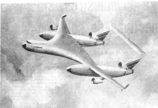
AVION DE CARGA DE FUSELAJES MULTIPLES.- Los ingenieros de la compañía estadounidense Lockheed-Georgia, están considerando varias configuraciones para sus nuevas aeronaves, incluyendo una con tres secciones de fuselajes separadas y un peso bruto de medio millón de libras. La carga útil del avión sería de 441.000 libras, con el 50% ubicada en el fuselaje central y el 25% en cada una de las secciones exteriores. (CPS).
