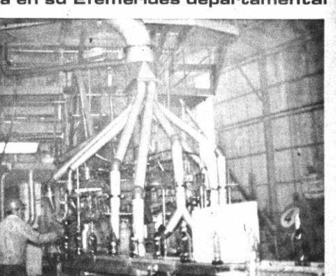
Máquina soplabra automática en plena producción de envases de vino tipo Burdeos y Borgoña simultáneamente. Se observa también el sistema de ventilación.
